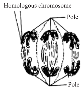
Fig. 4.15g Anaphase
